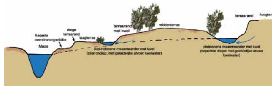
Kwelsituaties langs de Zandmaas (terrassenrivier).
