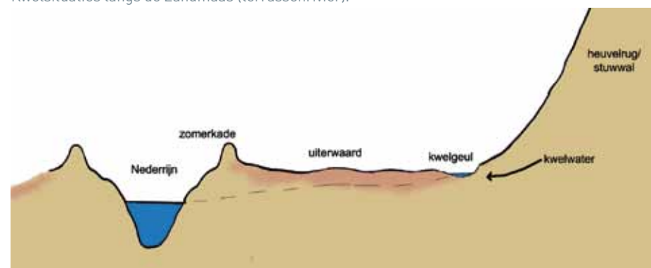
Kwelsituatie langs de Nederrijn (laaglandrivier langs heuvelrug).
